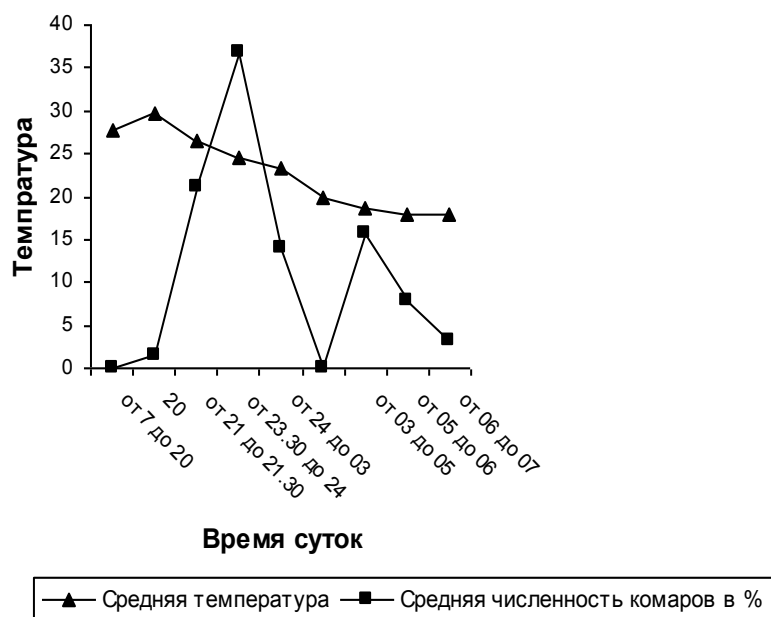
Рис. 2. Схема суточной ритма активности Anopheles maculipennis Mg. в летний период (с 20 VII по 26 VIII, пос. Белиджи, 2005 г.)
