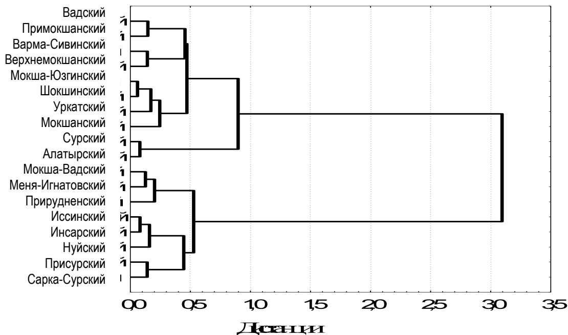
Рис. 2. Кластерная классификация пейзажных ареалов по признакам эстетичности (метод Варда)
