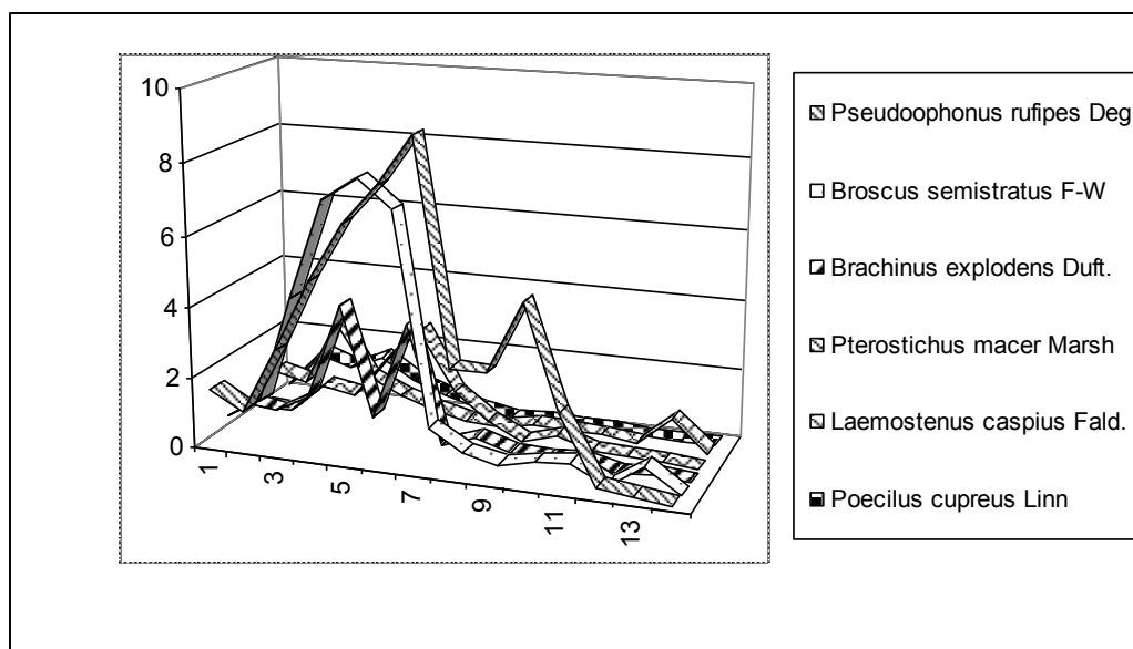
Рис. 2. Суммарный график сезонной динамики численности жукелиц.
