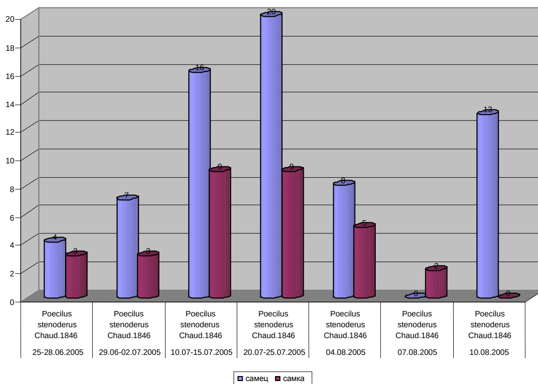
Рис. 2. Сезонная динамика Poecilus stenoderus Chaud. хребта Нукатль
