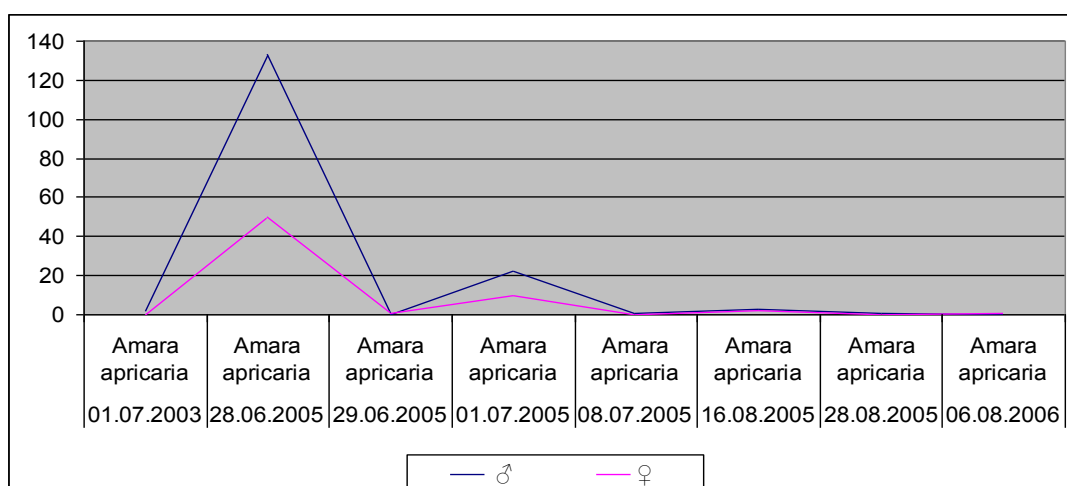
Рис. 2. Сезонная динамика жуужелиц вида Amara apricaria Тляратинского района (2005 г.)
