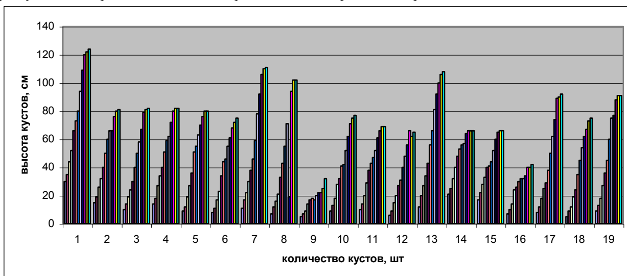
Рис. 2. Динамика роста семенных растений в открытом грунте
