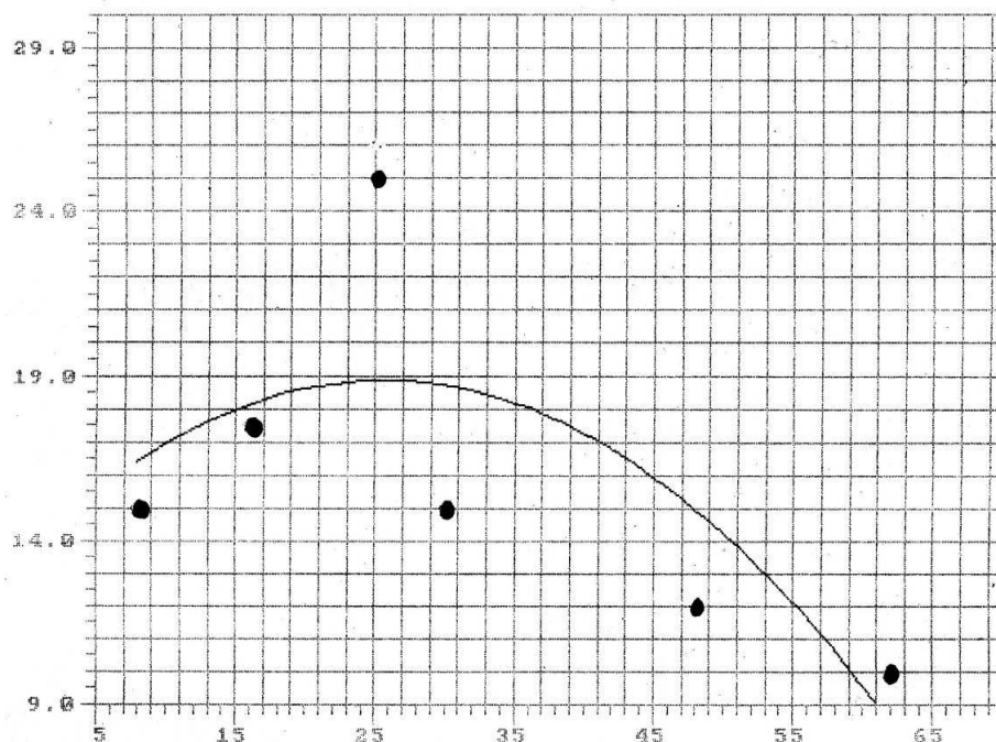
Рис.1. Изменение концентрации глюкозы в водных вытяжках из мышц молоди тилляпии в течении эксперимента
