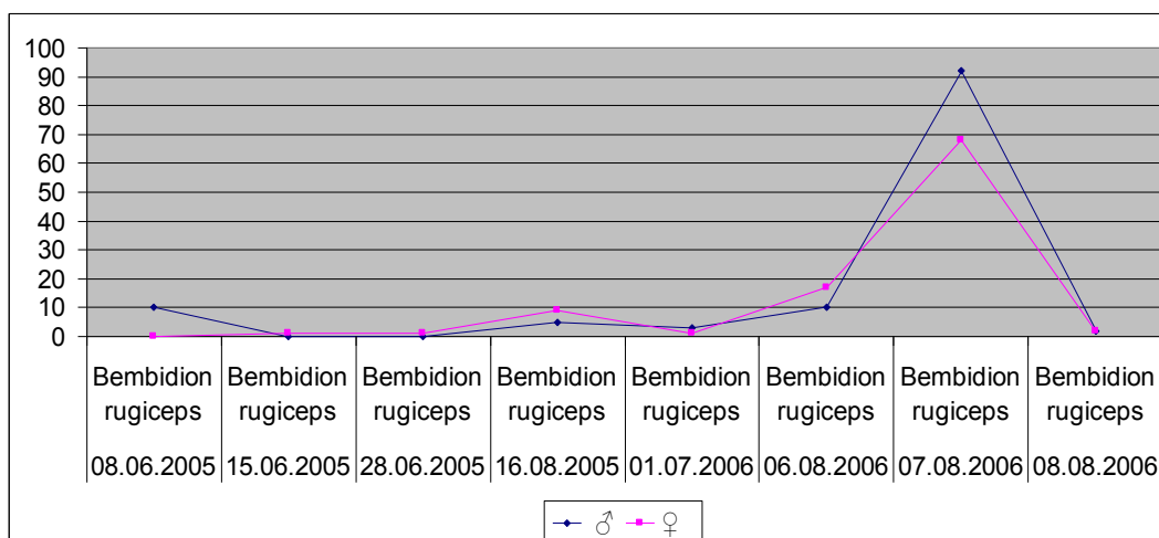
Рис.3. Сезонная динамика жукелиц вида Bembidion rugiceps Тлярятинского района (2005 г.)
