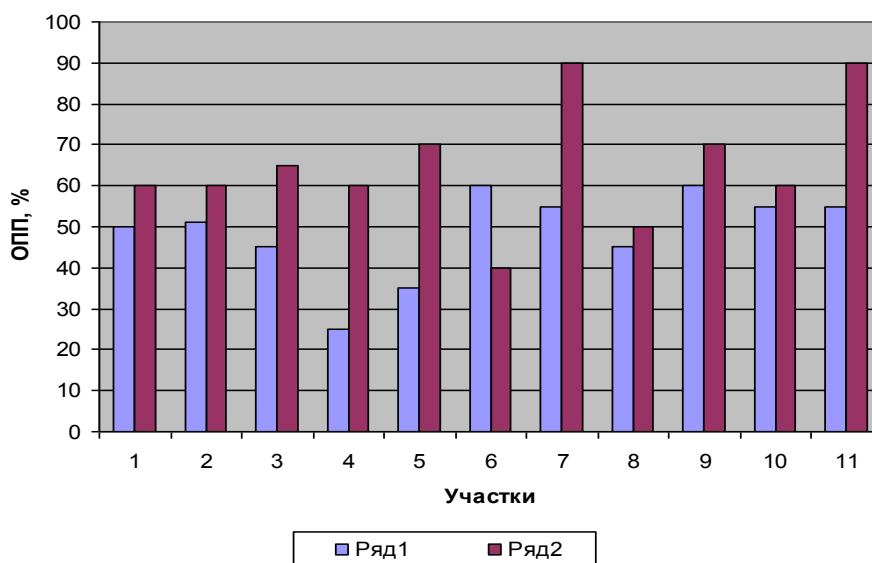
Рис. 1. Общее проективное покрытие фитомассы
