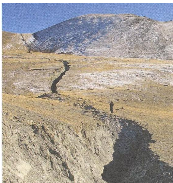
Рис. 1. Сейсморвы в урочище Узюк [5]
