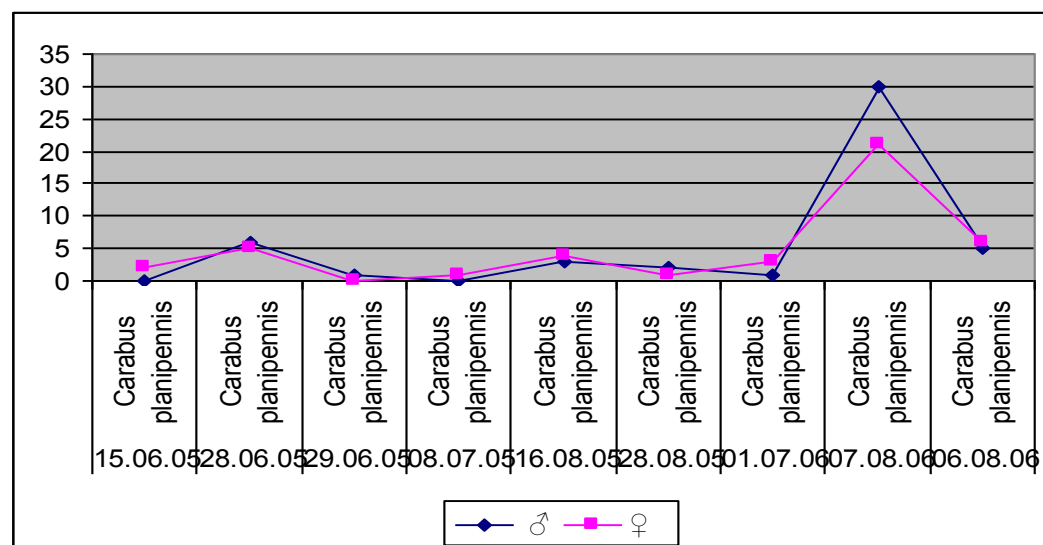
Рис.5. Сезонная динамика жукелиц вида Carabus planipennis Тлярятинского района (2006 г.)
