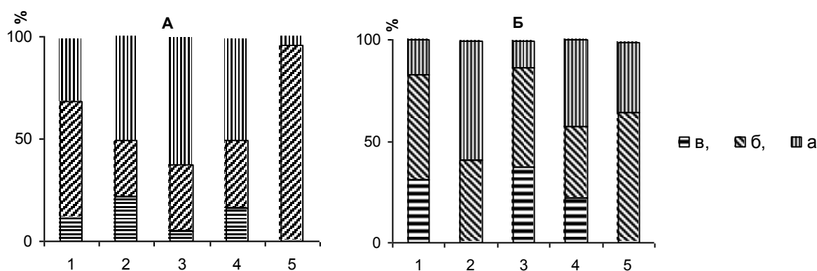
Примечание: длина корня и побега фасоли, подсолнечника, пшеницы, акации и гледичии (1 - 5). Обозначения: контроль (а), 20, 50 мл буровой смеси на 100 мл воды (б, в)
