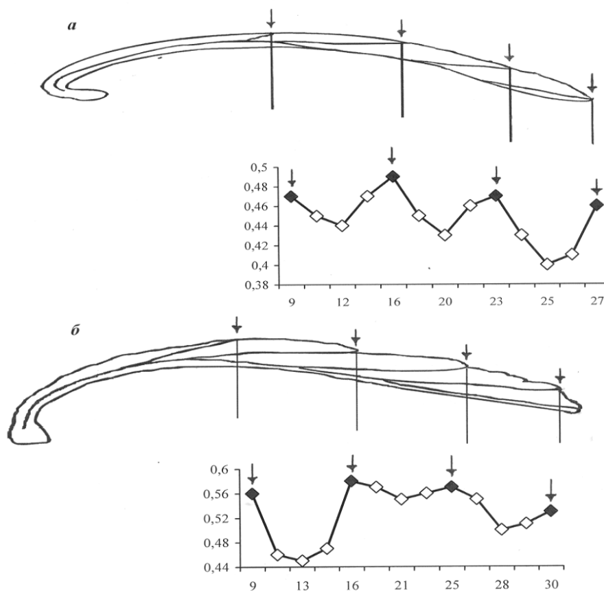
Рис. 2. Сезонные и онтогенетические колебания стронция у моллюсков:
