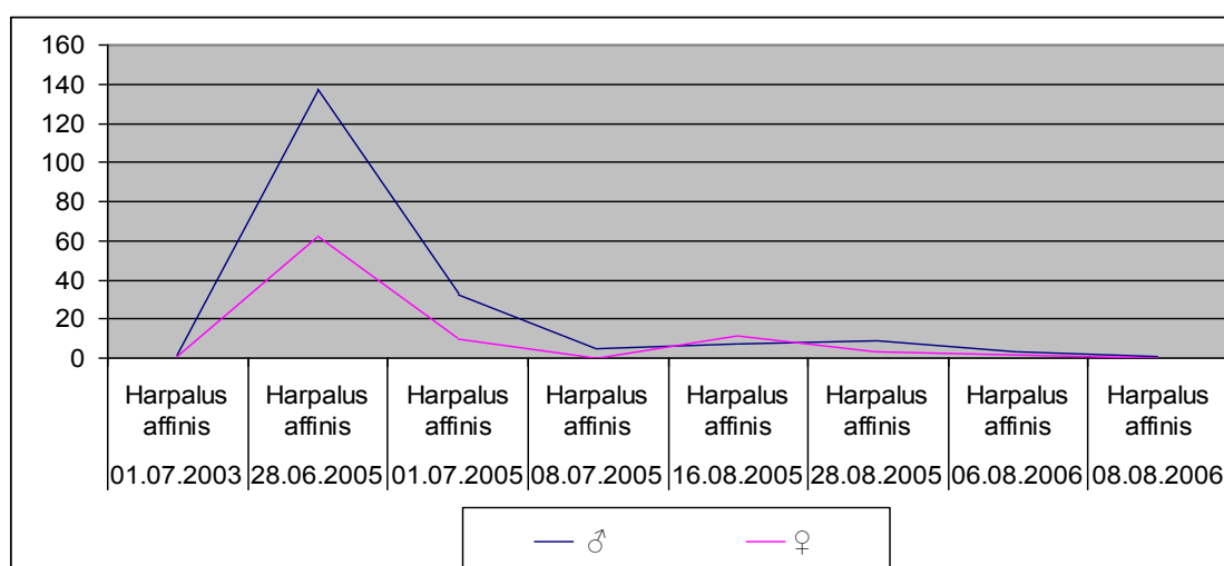
Рис.1. Сезонная динамика жуужелиц вида Harpalus affinis Тляратинского района (2003 г.)
