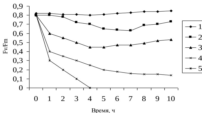
Рис. 1. Влияние \text{Cu}^{2+} в концентрации К(1), 10(2), 20(3), 40(4), 60(5) \text{мкг/л} на изменения переменной флуоресценции F_v/F_m микроводорослей Каспия при освещении 30 \text{ Вт/м}^2 .
