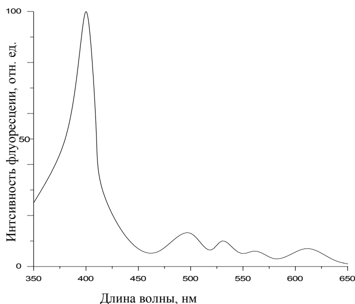
Рис. 4. Спектр возбуждения флуоресценции этилацетатного экстракта из изолированных плазматических мембран ( \lambda_{\text{возб}}=675 \text{ нм} )
