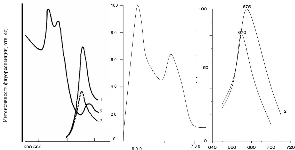
Рис. 1. Спектры флуоресценции изолированных плазматических мембран (1,2) и целых клеток (3) при возбуждении светом длиной волны 410 нм (1,3) или 280 нм (2). По оси ординат – интенсивность флуоресценции (I, отн.ед.), по оси абсцисс – длина волны ( \lambda , нм).
