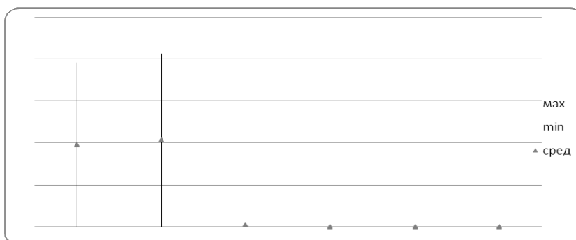
Рис. 16. Изменение содержания Zn в северной части Аграханского залива за весь период исследований
