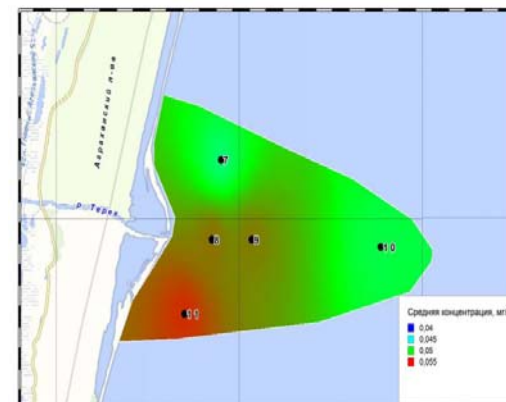
Рис. 5 Средняя концентрация НУ в морской воде в июле, мг/л, в районе взморья р. Терек [5] Fig. 5 The average concentration of oil hydrocarbons in the seawater in July, mg / l, in the seaside district of the Terek River [5]
